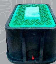
Barrenos ciegos en ambos costados de Ø7 cm
