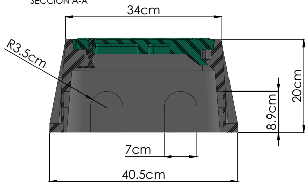
SECCIÓN A-A
